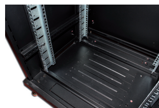
4 montants 19'' ajustables
